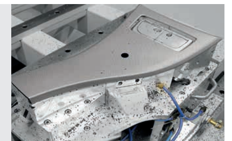
Spannvorrichtung mit Interieur-Bauteil auf einer ECO-NT.
