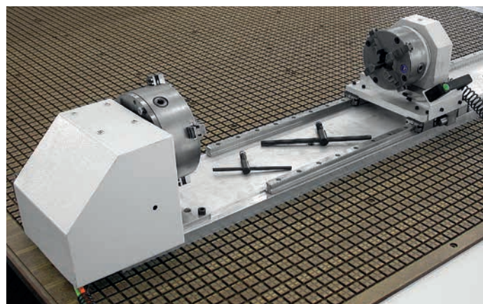
Kleine NC-Drehachse (bis Ø 310 mm) auf Vakuumrastertisch.
