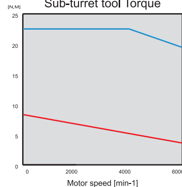
DT FANUC Sub-turret tool Torque
