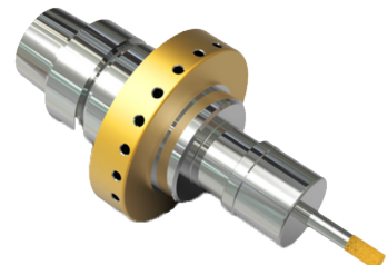
超声加工专用刀柄 Ultrasonic knife handle
