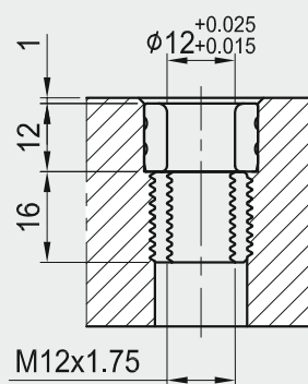
ø12 MTP hole
