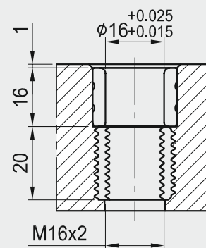
ø16 MTP hole
