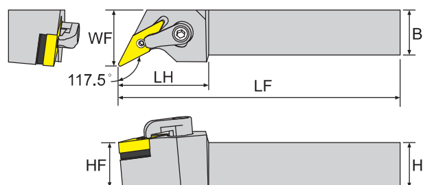
寸法 Dimension(mm)
