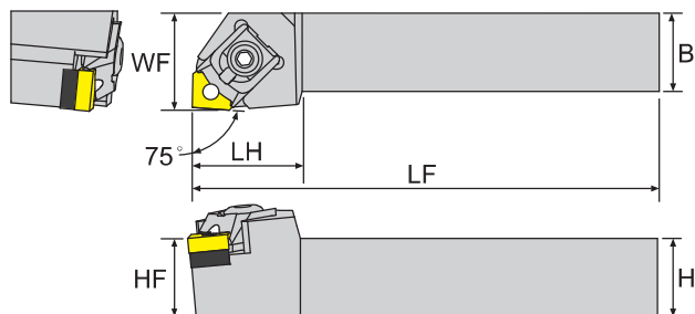
寸法 Dimension(mm)
