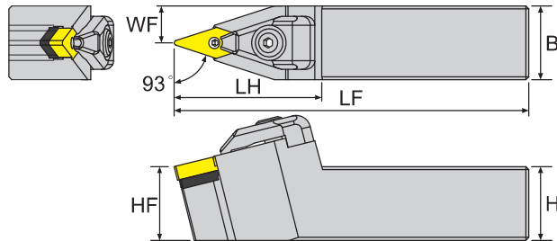
寸法 Dimension(mm)
