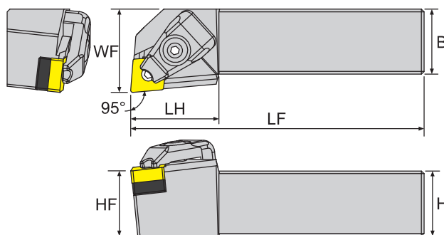
寸法 Dimension(mm)
