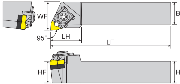
寸法 Dimension(mm)
