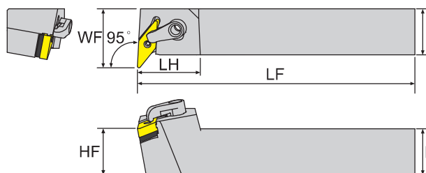
寸法 Dimension(mm)
