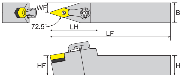
寸法 Dimension(mm)
