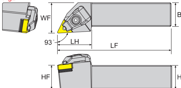
寸法 Dimension(mm)
