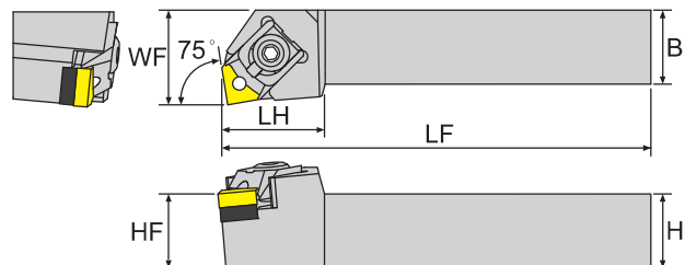
寸法 Dimension(mm)
