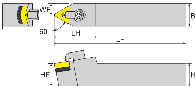
寸法 Dimension(mm)
