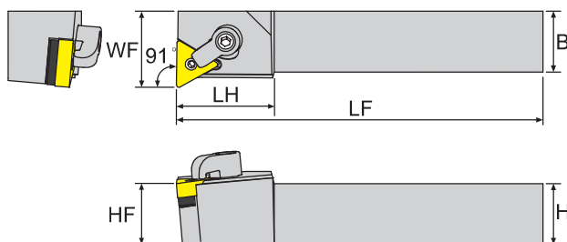
寸法 Dimension(mm)
