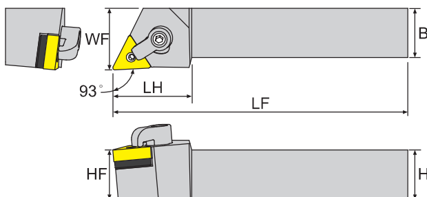
寸法 Dimension(mm)
