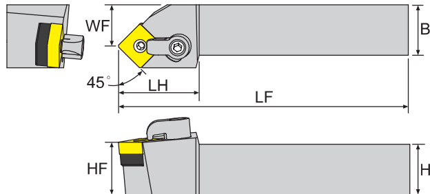
寸法 Dimension(mm)
