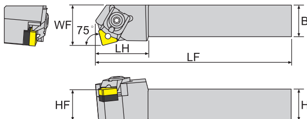
寸法 Dimension(mm)
