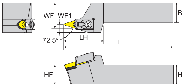
寸法 Dimension(mm)
