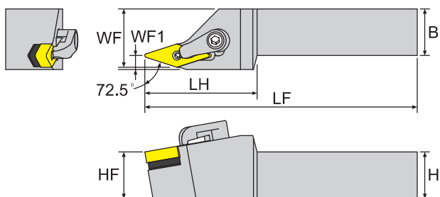
寸法 Dimension(mm)
