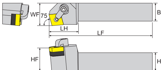
寸法 Dimension(mm)
