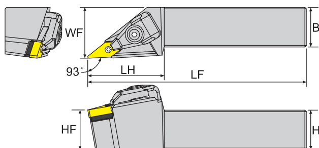
寸法 Dimension(mm)
