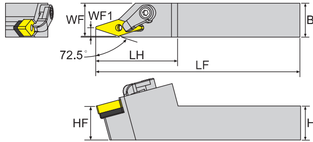
寸法 Dimension(mm)
