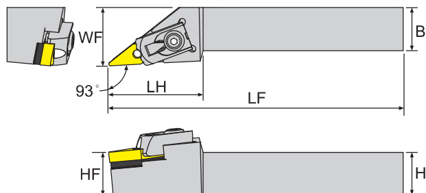
寸法 Dimension(mm)
