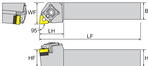
寸法 Dimension(mm)
