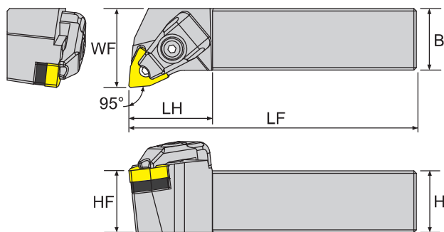
寸法 Dimension(mm)
