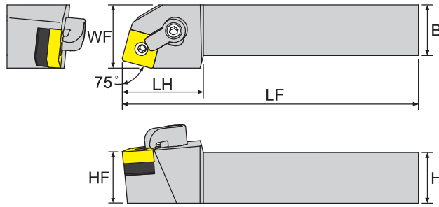
寸法 Dimension(mm)
