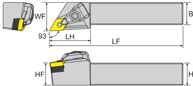
寸法 Dimension(mm)
