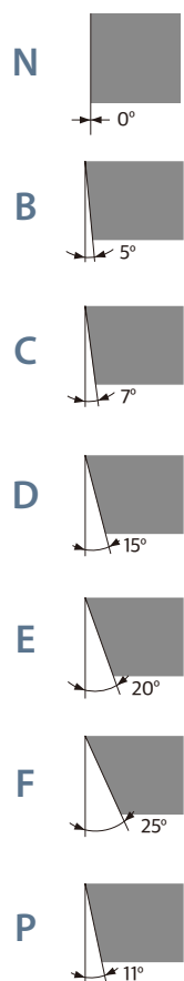
② Relief angle 主切削刃后角
